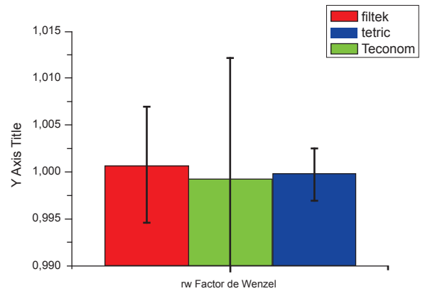
Gráfico 5. Factor de Wenzel para las resinas compuestas Filtek Z 250, Tetric Ceram y Te Econom.
